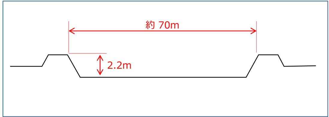
＜ 発寒遊水地（右岸）標準断面図（追加支援箇所）＞
